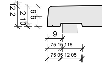
Dak ronding 1 : 10
